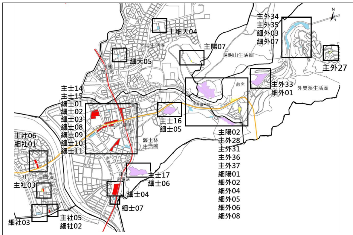
士林區細部計畫變更示意圖
