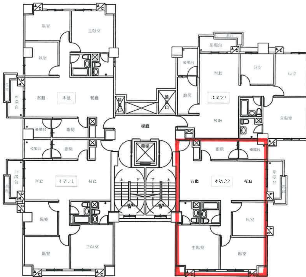
永平社會住宅 2、2-1、2-2、2-3 號標準層平面圖
